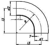
CODO 90° S. EXTRA LARGO EXTRA LONG WELD.BEND 90° ОТВОД УДЛИНЁННЫЙ 90° ПОД СВАРКУ
