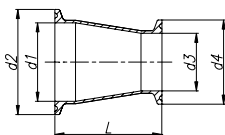
REDUC. CONCÉNTRICA CL/CL CONC. REDUCER CL/CL ПЕРЕХОД КОНИЧЕСКИЙ CL/CL
