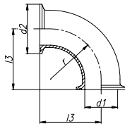
CODO 90° CL/CL BEND 90° CL/CL ОТВОД 90° CL/CL
