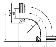
CODO 90° M/M SMS BEND 90° M/M SMS ОТВОД SMS 90° НАРУЖ.РЕЗЬБА/ НАРУЖ.РЕЗЬБА
