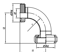
CODO 90° M/T SMS BEND 90° M/N SMS ОТВОД SMS 90° НАРУЖ.РЕЗЬБА/ГАЙКА
