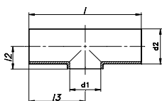
TE SOLDAR CORTA SMS SHORT WELDING TEE SMS ТРОЙНИК КОРОТКИЙ SMS ПОД СВАРКУ
