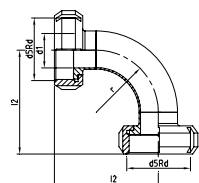
CODO 90° T/T SMS BEND 90° N/N SMS ОТВОД SMS 90° ГАЙКА / ГАЙКА
