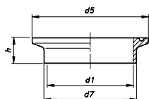
CASQUILLO CL SOLD. CORTO SHORT WELDING CLAMP ШТУЦЕР КОРОТКИЙ CLAMP ПОД СВАРКУ
