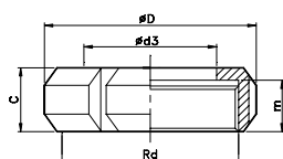
TUERCA SMS NUT SMS ГАЙКА SMS
