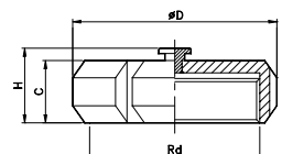
TUERCA CIEGA CON PIVOTE BLIND NUT WITH BOSS ГАЙКА-ЗАГЛУШКА С БОБЫШКОЙ
